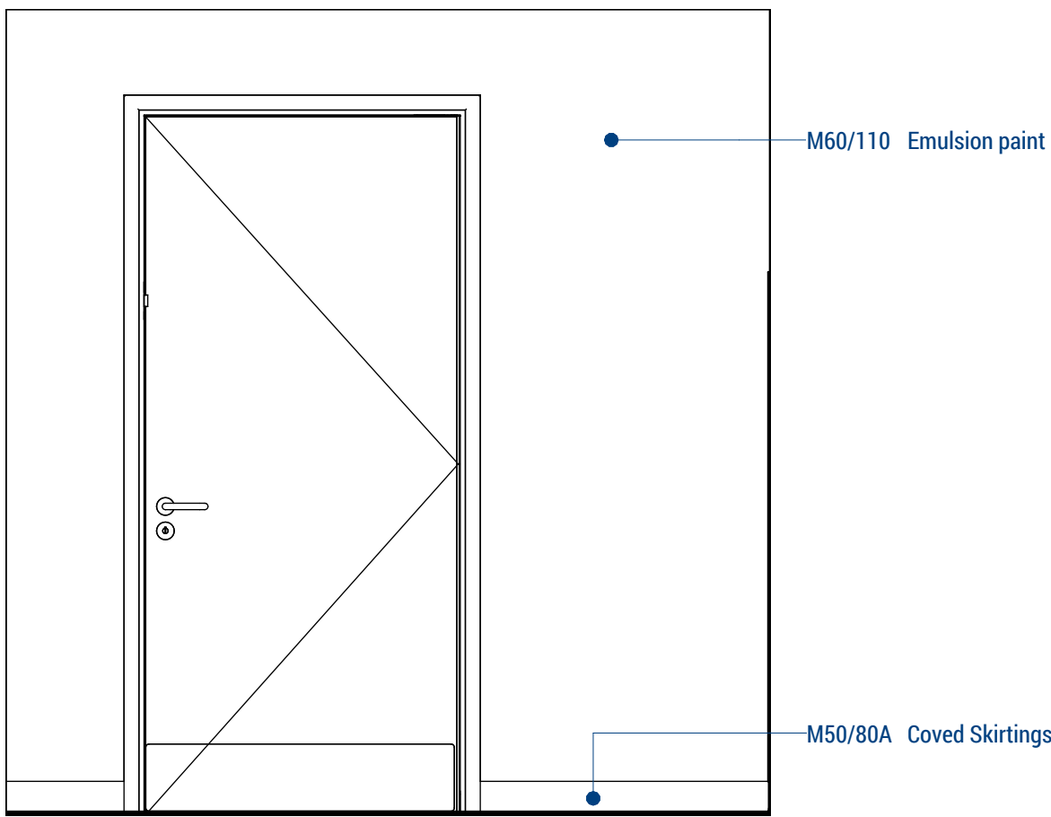
5. Acc WC 1 1 : 20
