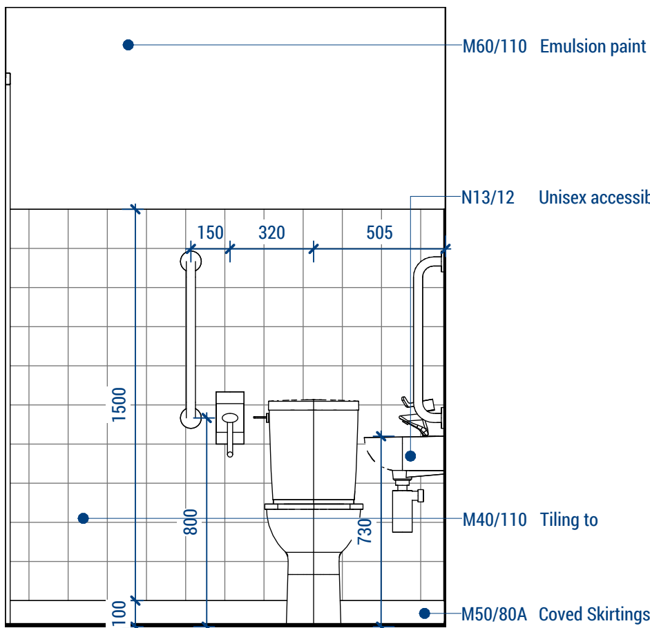
6. Acc WC 2 1 : 20
