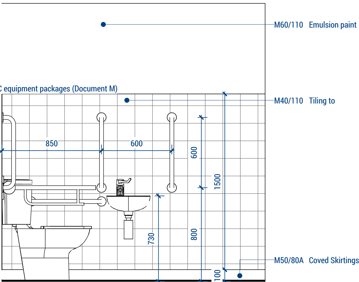
7. Acc WC 3 1 : 20
