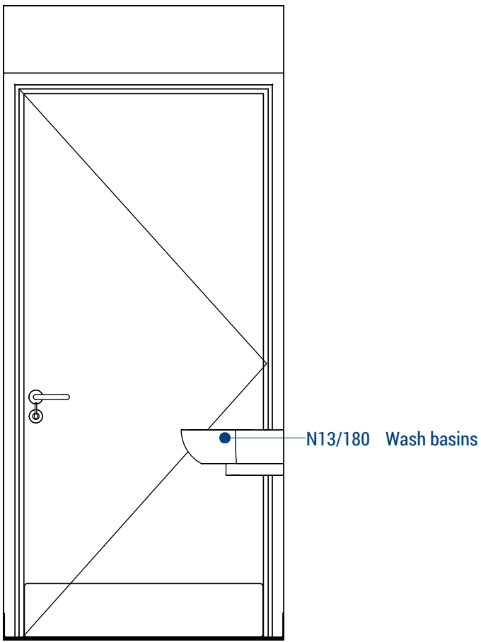
2. WC 2 1 : 20
