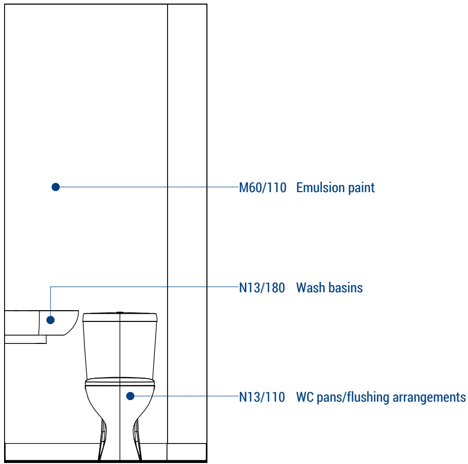
4. WC 4 1 : 20
