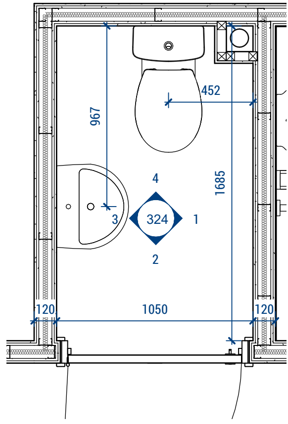
A. WC 1 : 20
