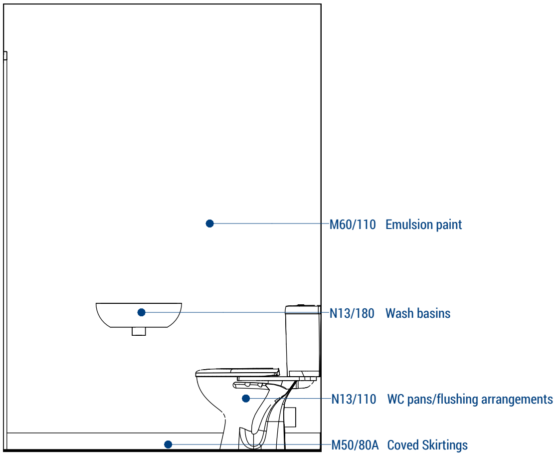
3. WC 3 1 : 20
