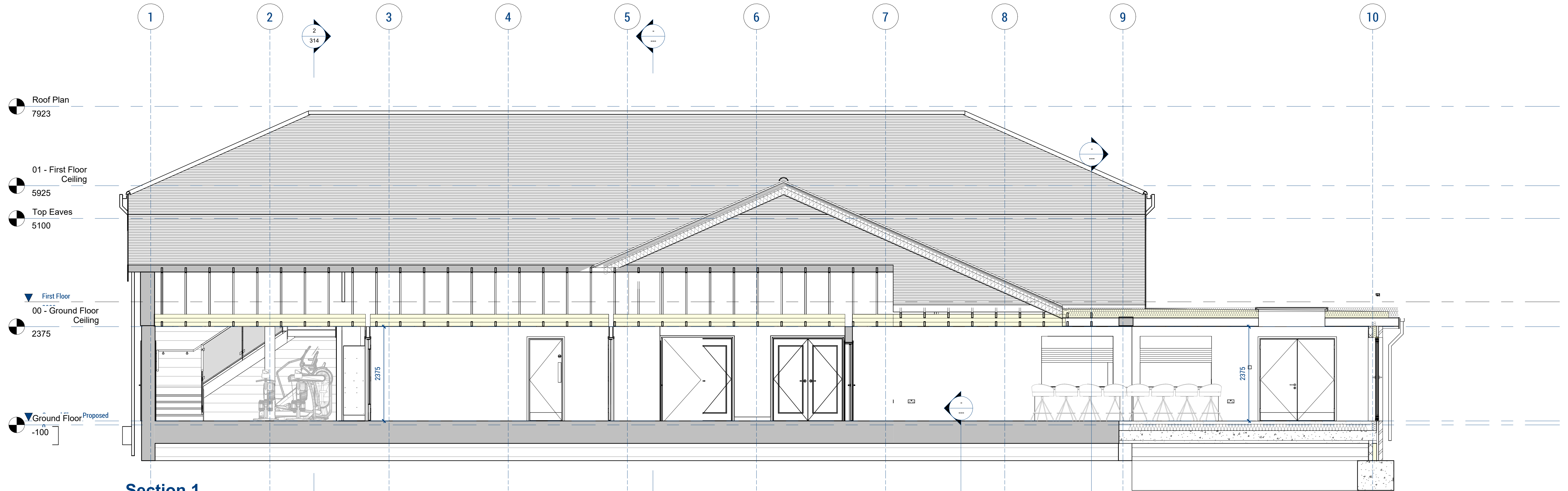
Section 1 1 : 50
