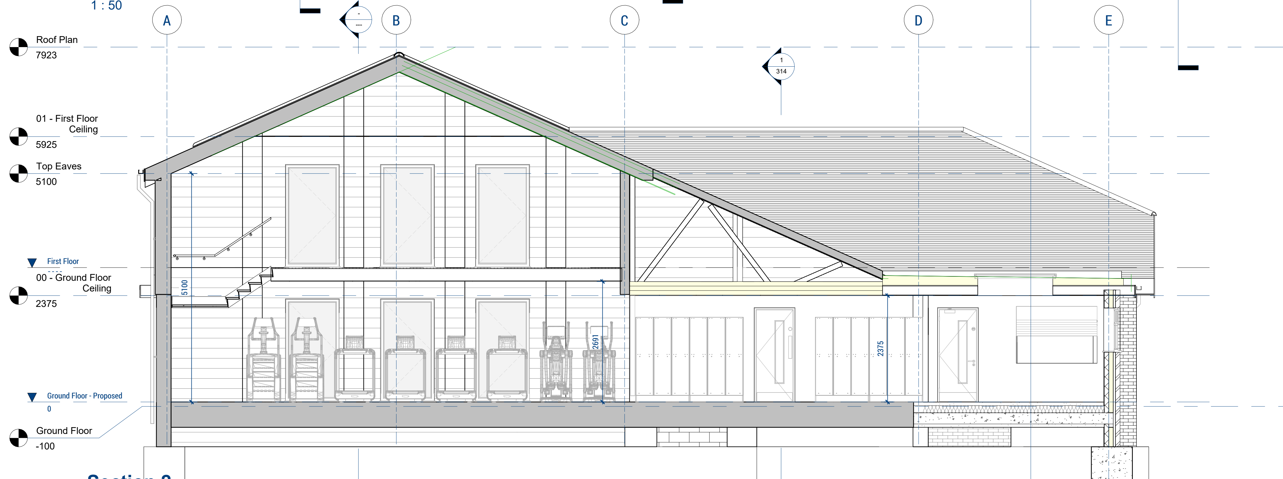
Section 2 1 : 50
