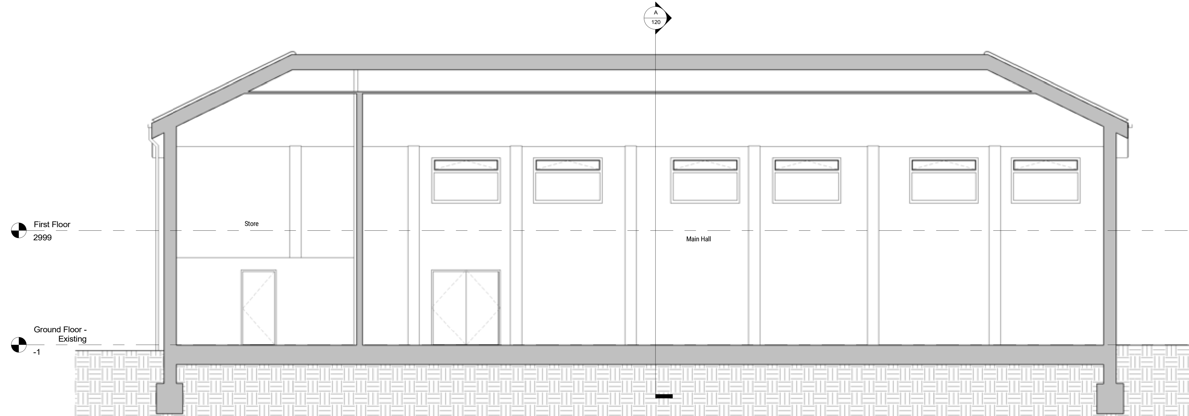
Section A - Existing 1 : 50
