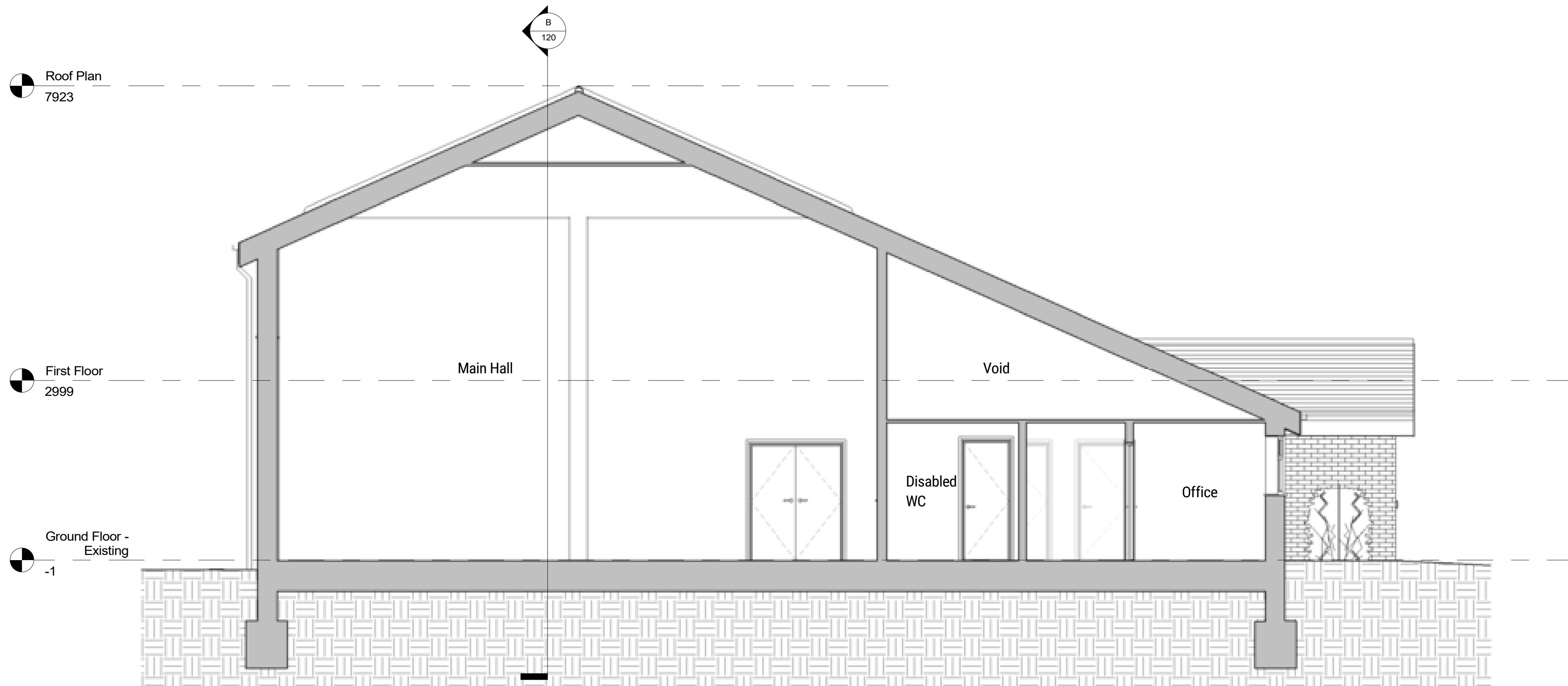
Section A - Existing 1 : 50
